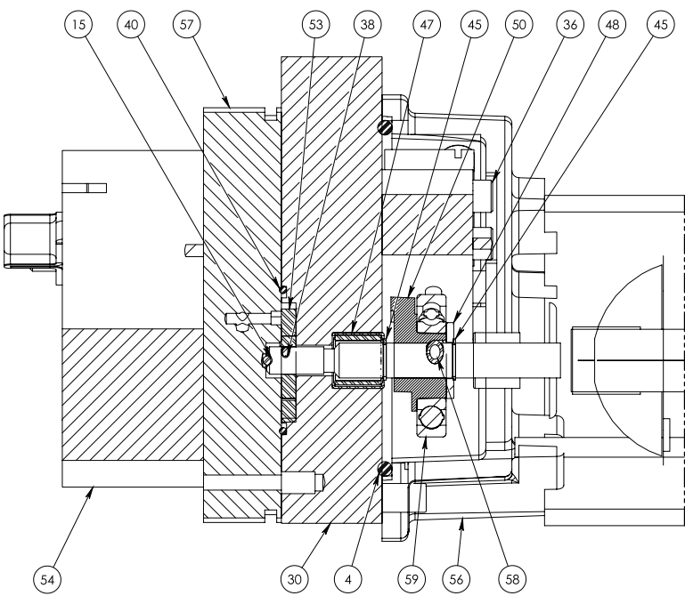
SECTION D-D
