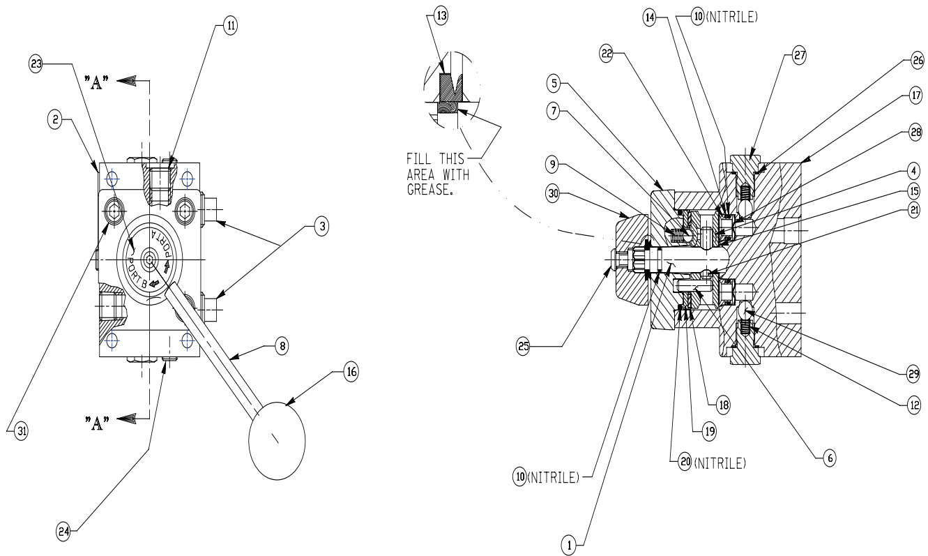
SECTION A-A
