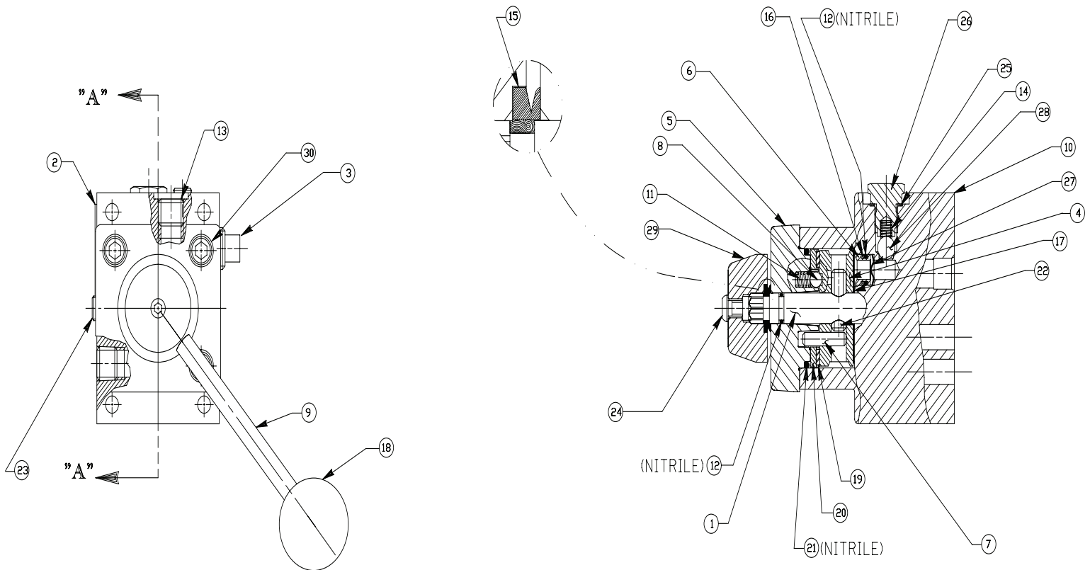
SECTION A-A
