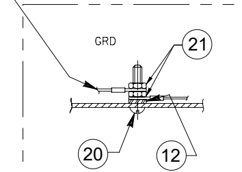
VIEW A-A
