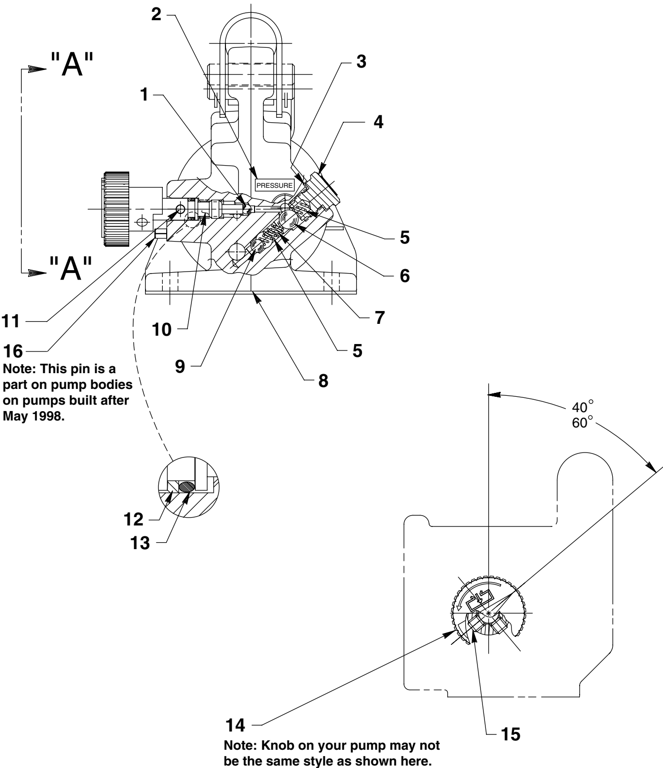
VIEW A-A
